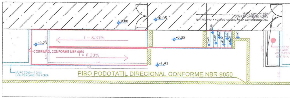
3 DETALHE DA RAMPA SEM ESCALA
