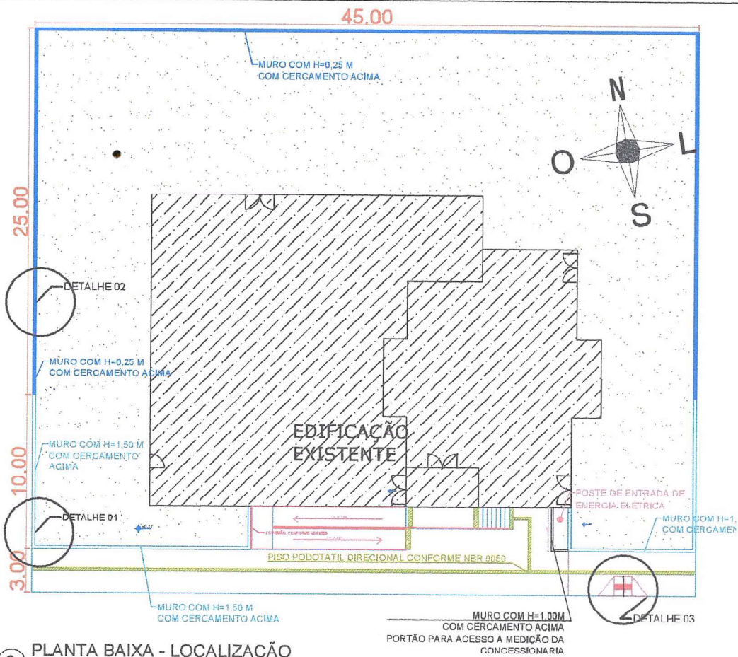
2 PLANTA BAIXA - LOCALIZAÇÃO 1:250
