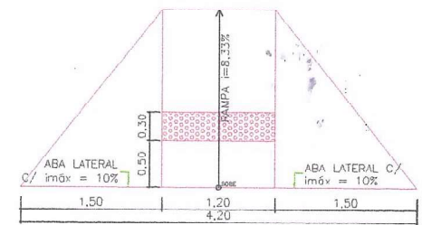
DETALHE DE REBAIXO DE MEIO FIO P/ PEDESTRES DETALHE 03
